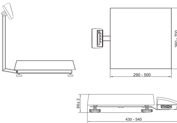
Konstrukce váhy WTC/C
